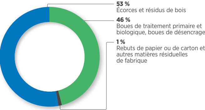
Figure 1.2 MATIÈRES RÉSIDUELLES DES PAPETIÈRES UTILISÉES EN COMBUSTION
