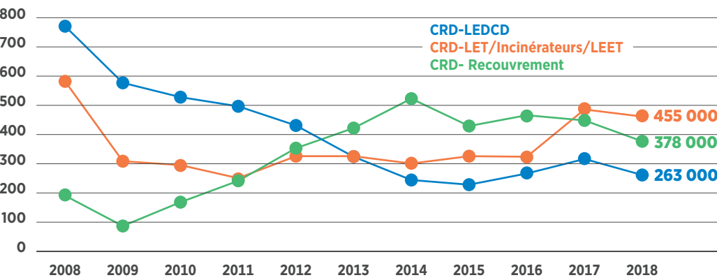
Figure 1.2 QUANTITÉ DE RÉSIDUS DE CRD UTILISÉS EN RECOUVREMENT OU AUTRES USAGES ET ÉLIMINÉS DANS LES DIFFÉRENTS LIEUX (en milliers de tonnes)
