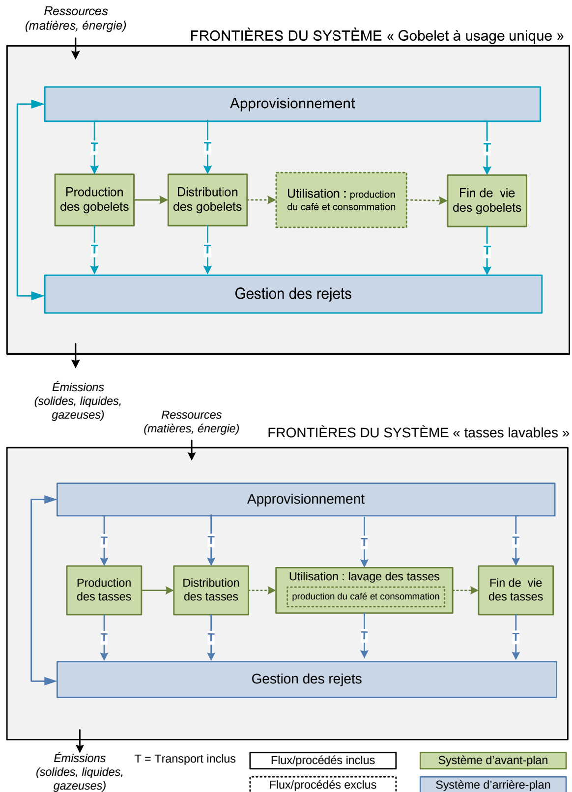
Figure 2-2 : Frontières des systèmes de gobelets à usage unique (haut) et tasses lavables fournies par le restaurateur ou par le client (bas).
