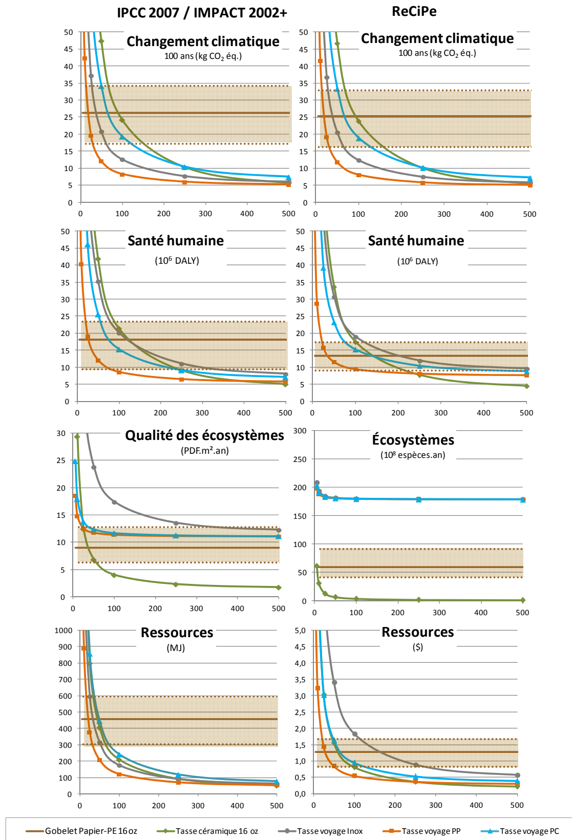
Figure 3-3 : Comparaison des options pour servir un café par jour pendant un an, selon les méthodes ReCiPe et IMPACT 2002+ / IPCC 2007.
