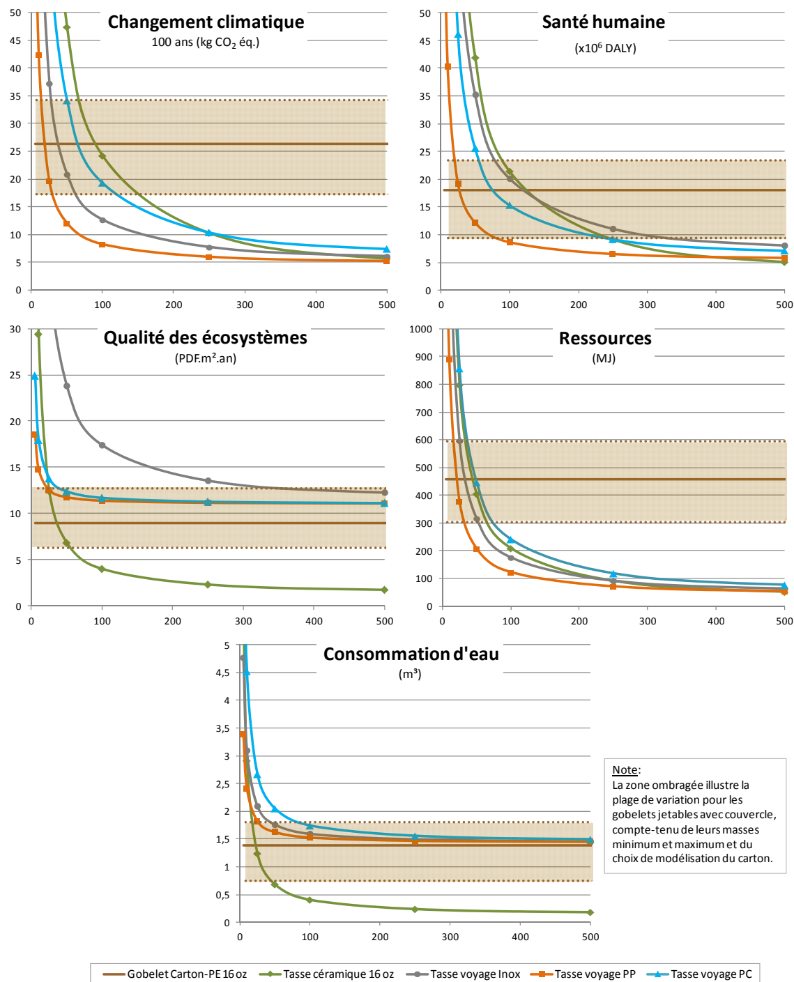
Figure 2: Comparaison de cinq options pour servir un café par jour pendant un an, en fonction du nombre de réutilisations des tasses (méthode IMPACT 2002+).
