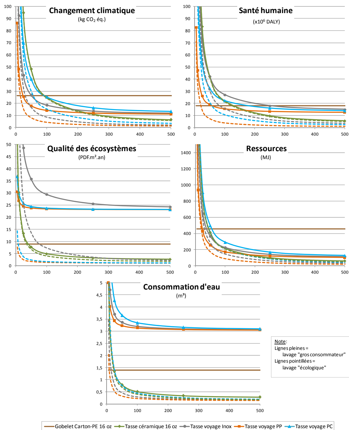
Figure E-1 : Comparaison de cinq options pour servir un café par jour pendant un an, en fonction du nombre de réutilisations des tasses (méthodes IMPACT 2002+ et IPCC 2007) – Analyse de sensibilité considérant des scénarios de lavage « gros consommateur » et « écologique ».
