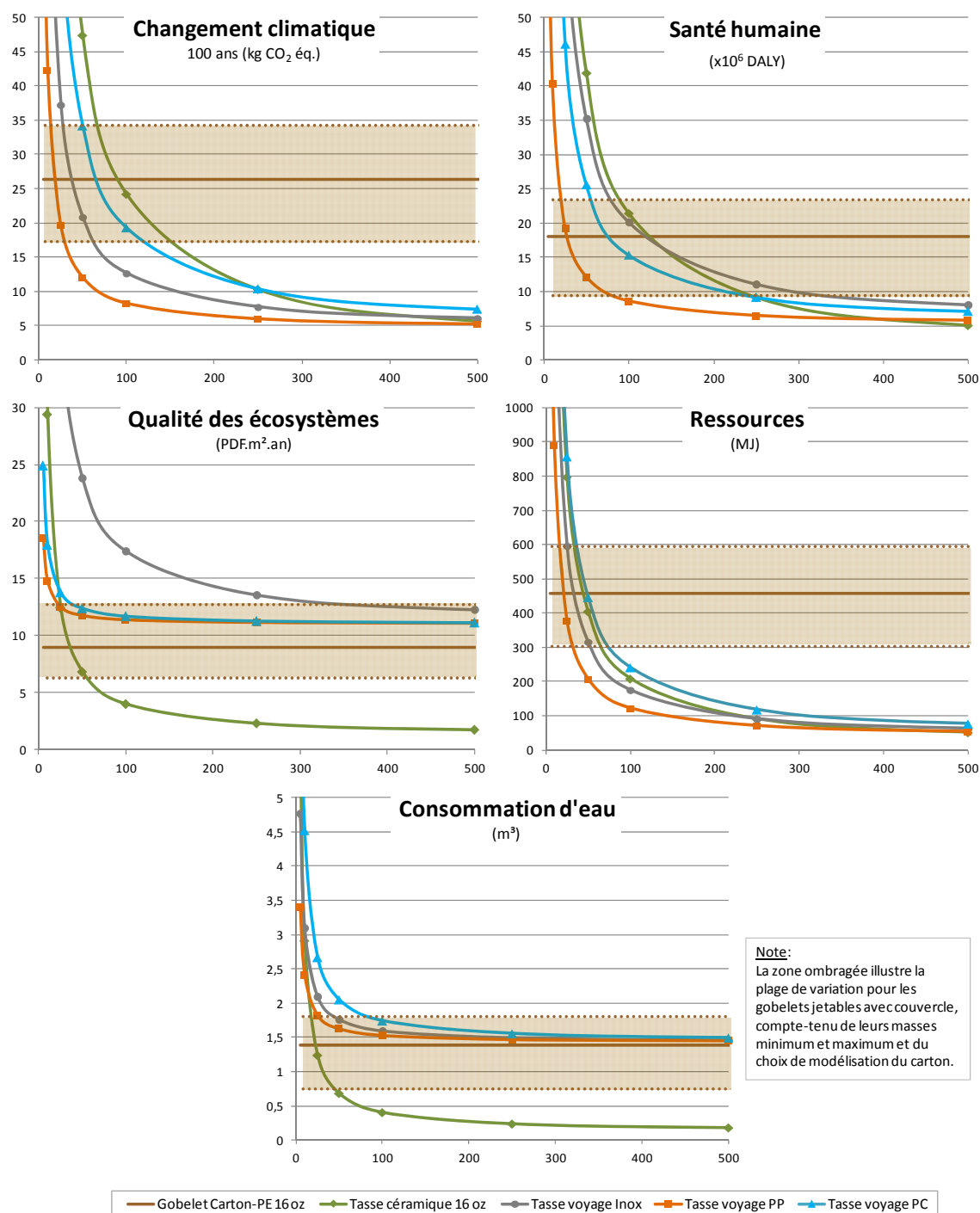
Figure 3-2 : Comparaison de cinq options pour servir un café par jour pendant un an, en fonction du nombre de réutilisations des tasses (méthodes IMPACT 2002+ et IPCC 2007).
