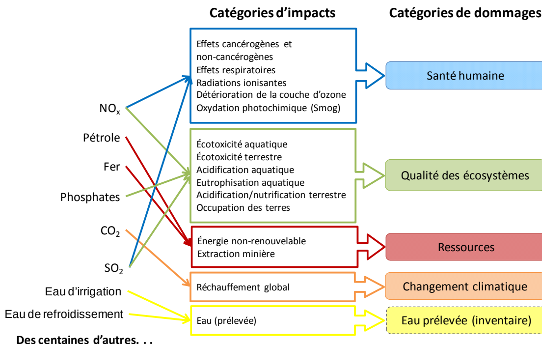
Figure 2-3 : Catégories de dommage et catégories d'impacts de la méthode IMPACT 2002+.
