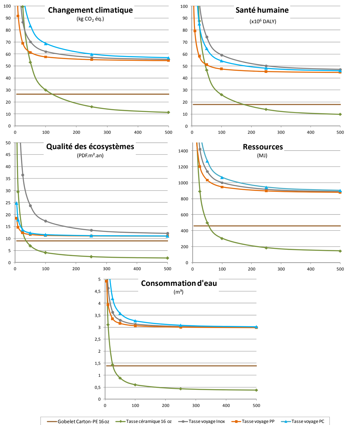
Figure E-2 : Comparaison de cinq options pour servir un café par jour pendant un an, en fonction du nombre de réutilisations des tasses (méthodes IMPACT 2002+ et IPCC 2007) – Analyse de sensibilité considérant un approvisionnement énergétique nord-américain moyen pour le lavage des tasses.
