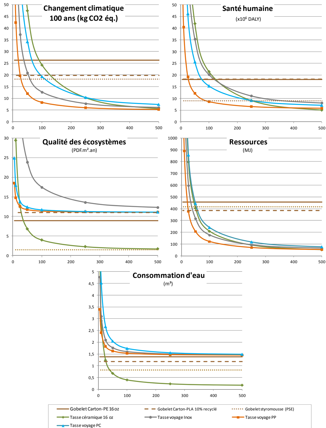
Figure 3-4 : Comparaison d'options pour servir un café par jour pendant un an, en fonction du nombre de réutilisations des tasses (méthodes IPCC 2007 et IMPACT 2002+) – Analyse de sensibilité avec les gobelets compostables et les gobelets jetables en styromousse.
