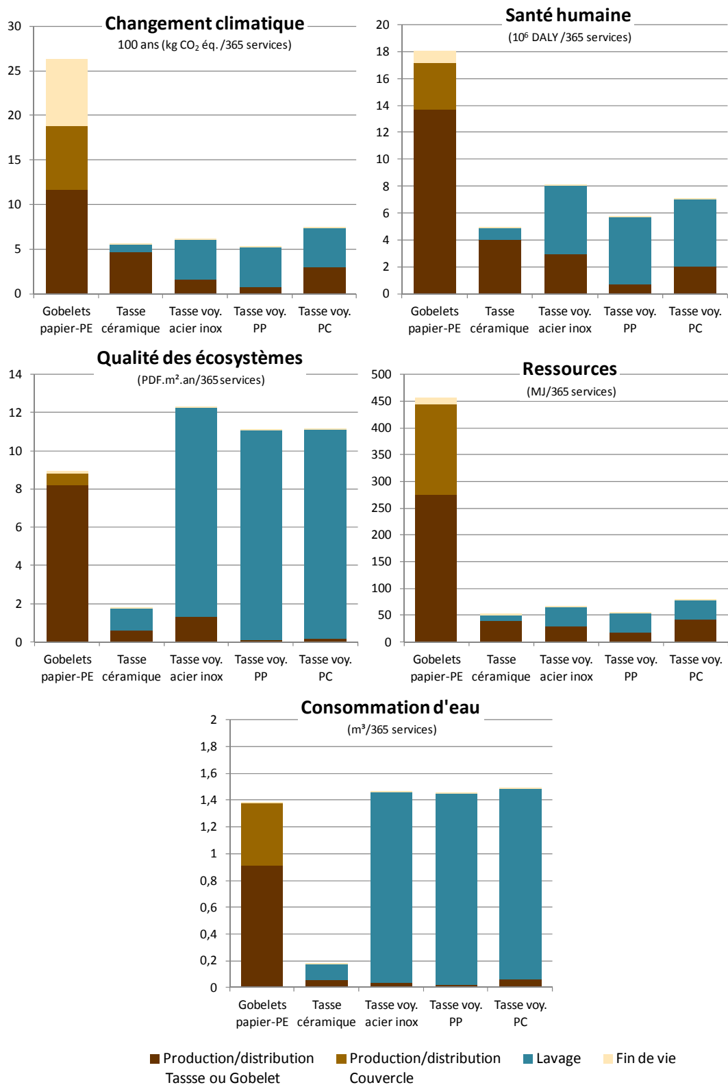
Figure 3-1 : Profil environnemental de cinq options pour servir un café par jour pendant un an (méthodes IMPACT 2002+ et IPCC 2007) (tasse en céramique et tasses de voyage réutilisées 500 fois).
